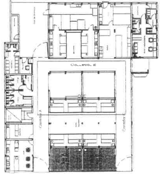
PLANTA FINAL
