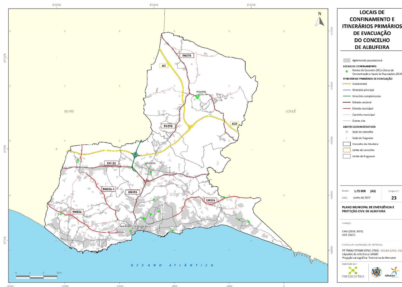
Carta 23. Locais de confinamento e itinerários primários de evacuação do concelho de Albufeira
