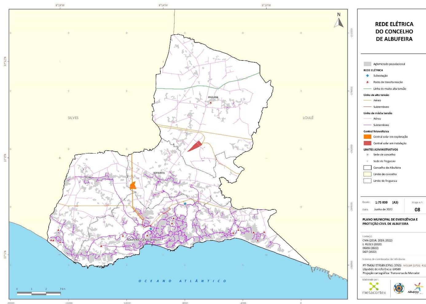
Carta 8. Rede elétrica do concelho de Albufeira
